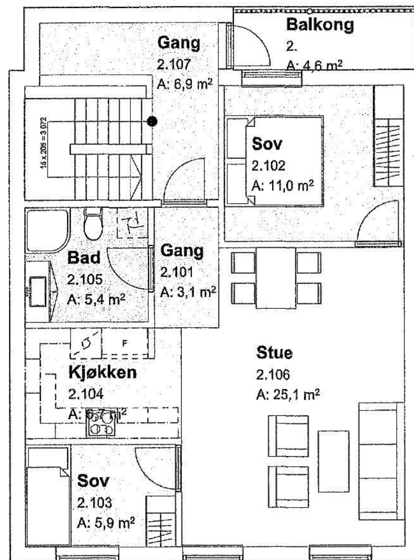
2 Etasje
